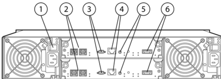
Dual Controller MSA2000fc G2
